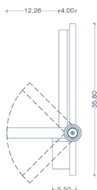
ELEVACIÓN LATERAL
