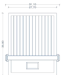
ELEVACIÓN POSTERIOR
