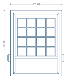
ELEVACIÓN FRONTAL
